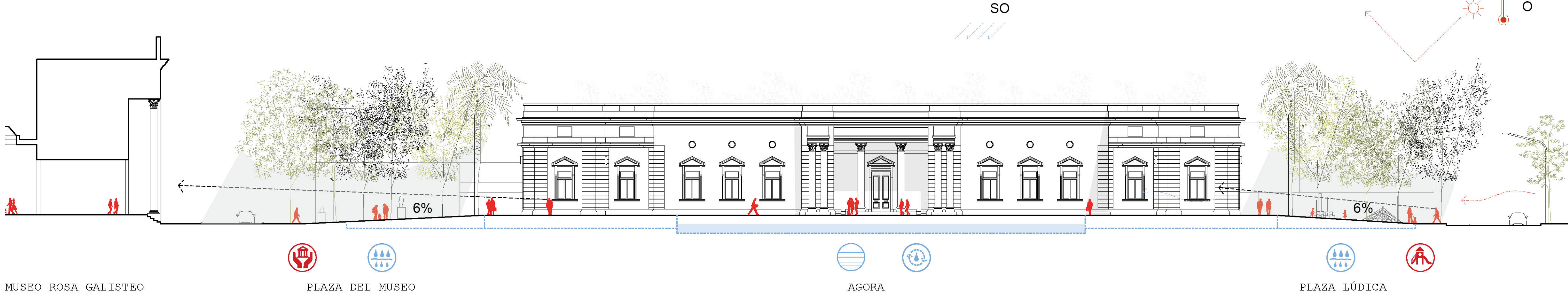
SECCION TRANSVERSAL. Escala 1:250
