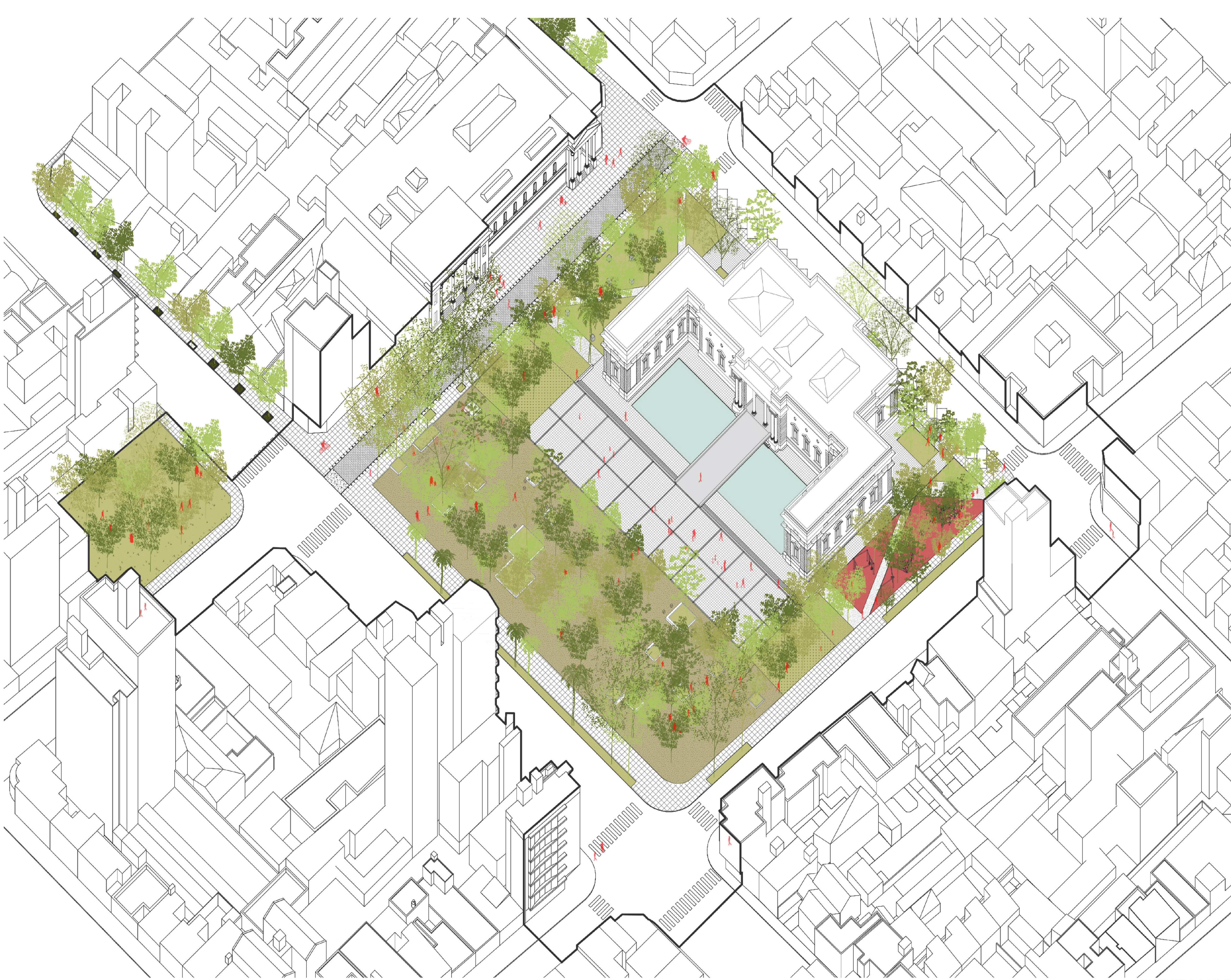
AXONOMETRIA
