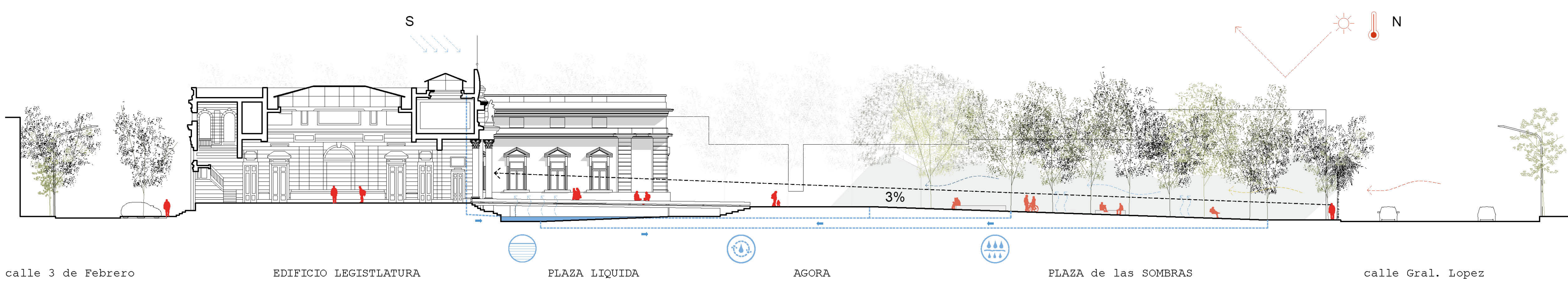
SECCION LONGITUDINAL. Escala 1:250
